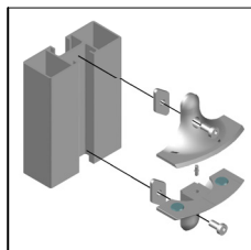
Montage des supports
